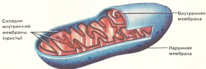
60. Схема строения митохондрии по данным электронного микроскопа.
