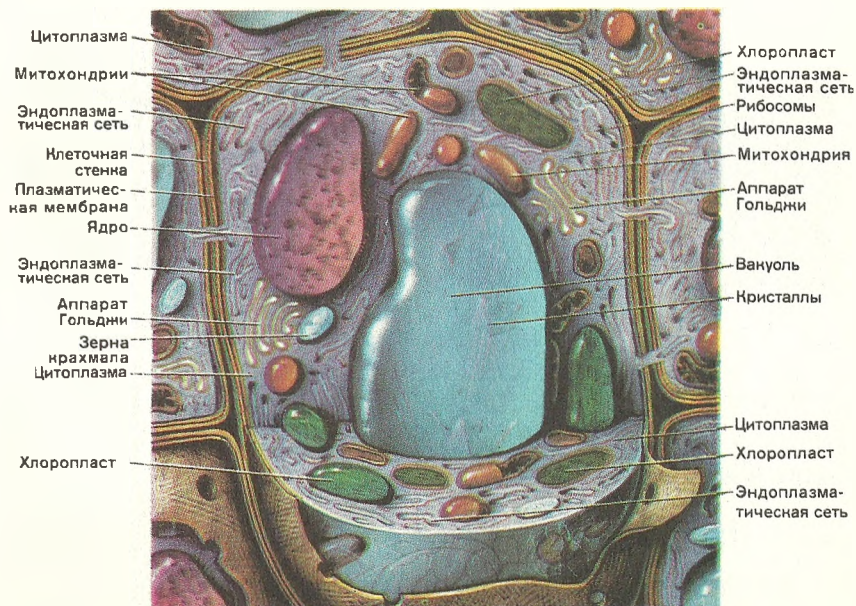
51. Схема строения растительной клетки по данным электронного микроскопа.
