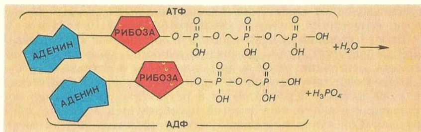
79. Структура АТФ. Превращение АТФ в АДФ ( \sim — макроэргическая связь).
