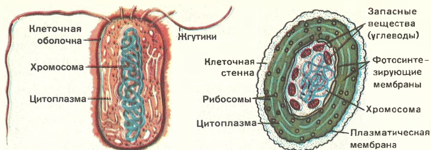
66. Схема строения бактерии (слева) и сине-зеленой водоросли (справа).
