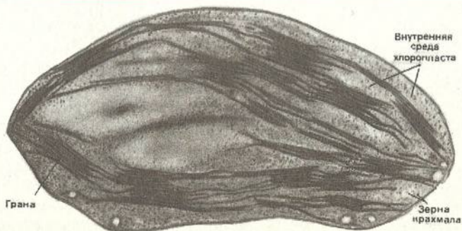
61. Электронно-микроскопическая фотография хлоропласта. Увел. 40 000.
