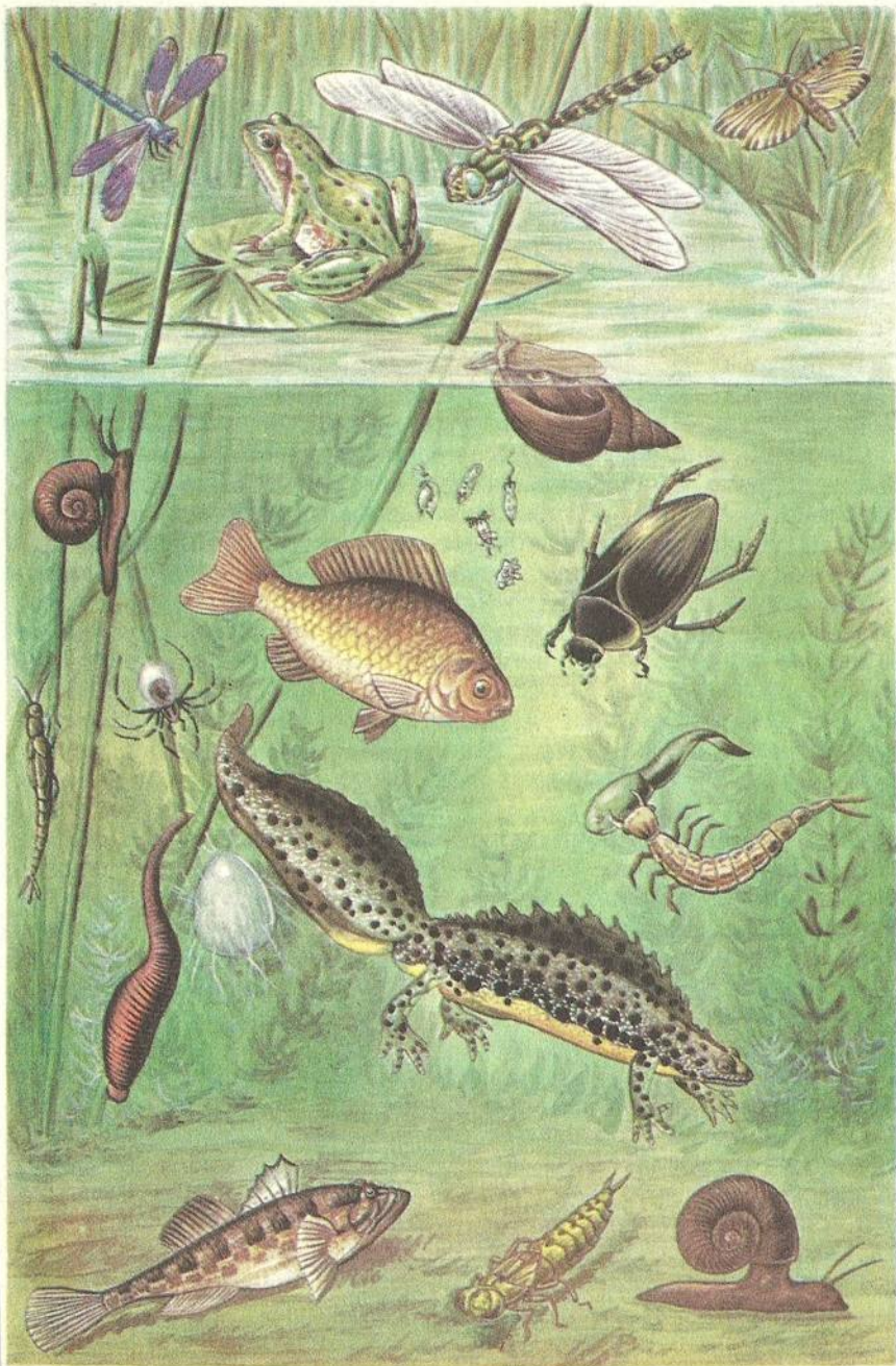
38. Биогеоценоз пресного водоема.
