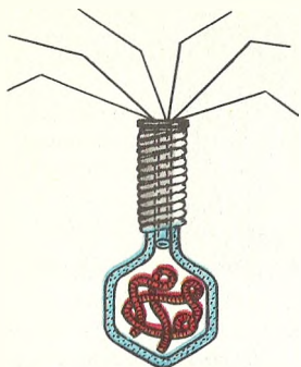
69. Схема строения бактериофага.
