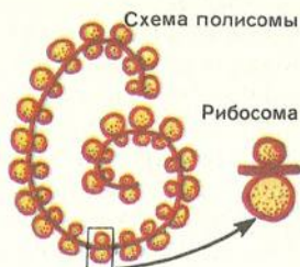
57. Гладкая эндоплазматическая сеть. 58. Электронно-микроскопическая фотография полисомы и схема полисомы и рибосомы.
