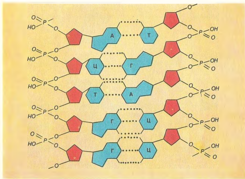
77. Участок двойной спирали ДНК.
