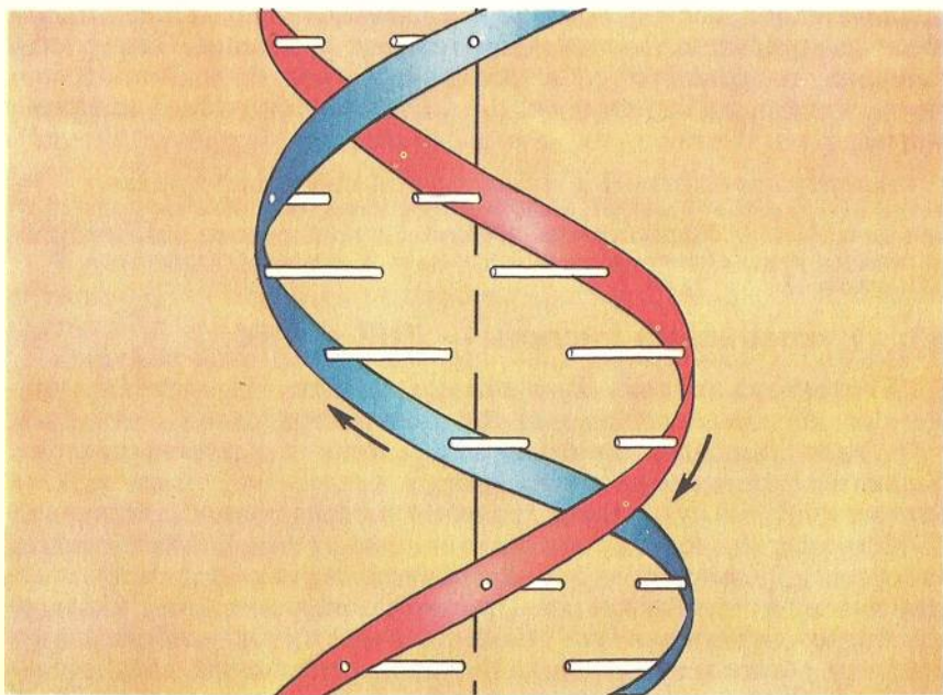
74. Схема строения ДНК (двойная спираль).
